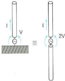
モノポール, ダイポール
