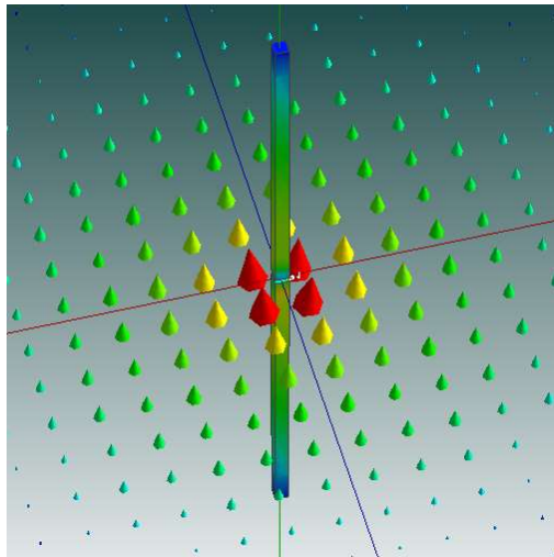
電界 E=(E_x,E_y,E_z)
