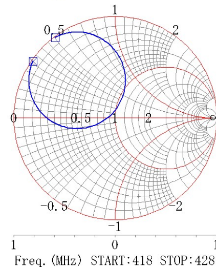
L: S11 □
