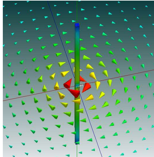
磁界 H=(H_x,H_y,H_z)
