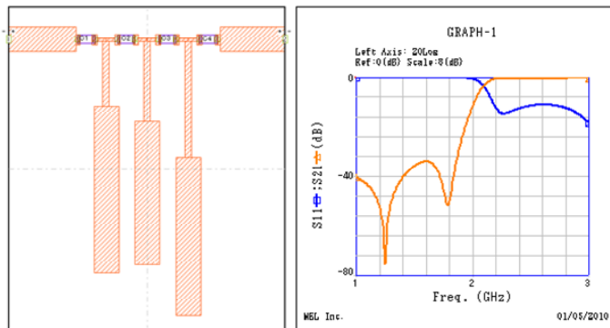
マイクロストリップ+キャパシタ
